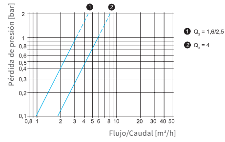
Curva de pérdida de presión
